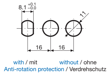
Cut-out Montageöffnung
